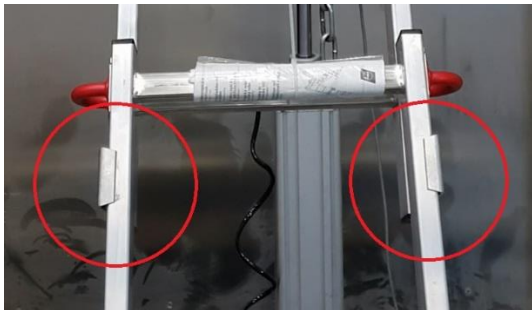
Die Schiebebeschläge umgreifen die Holme des unteren Leiterteils.
