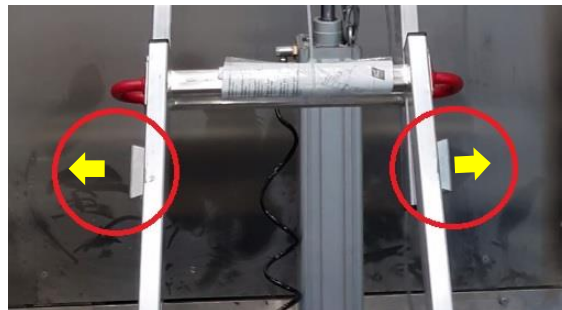
Die Schiebebeschläge biegen sich bei Belastung auf, die Leiter kollabiert.
